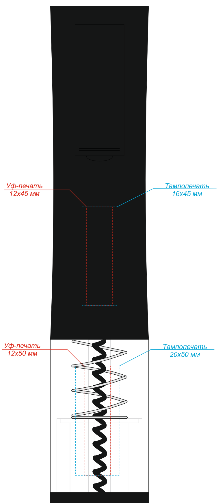
Вид сзади
